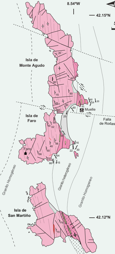
MAPA GEOLÓGICO DE LAS ISLAS CÍES
